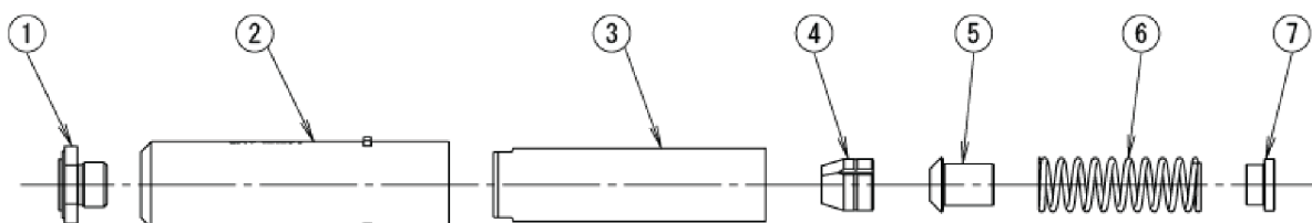
Fig. 6: Nose assembly AVSEAL 02964 16mm
